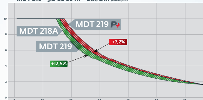
MDT 219 – jib de 65 m – SM/DM (exemplo)
