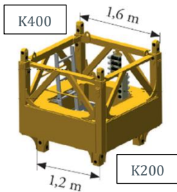
Elemento di raccordo inverso K20/K40
