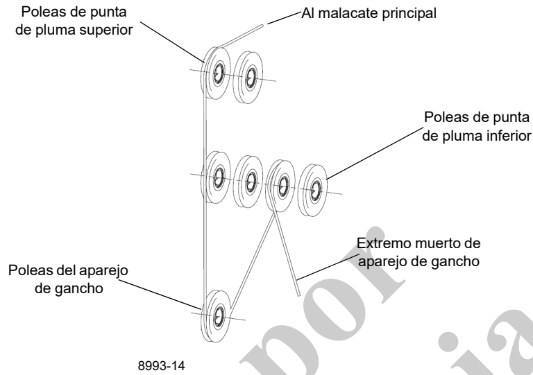
Cable de 3 secciones, aparejo de gancho con 1 polea
