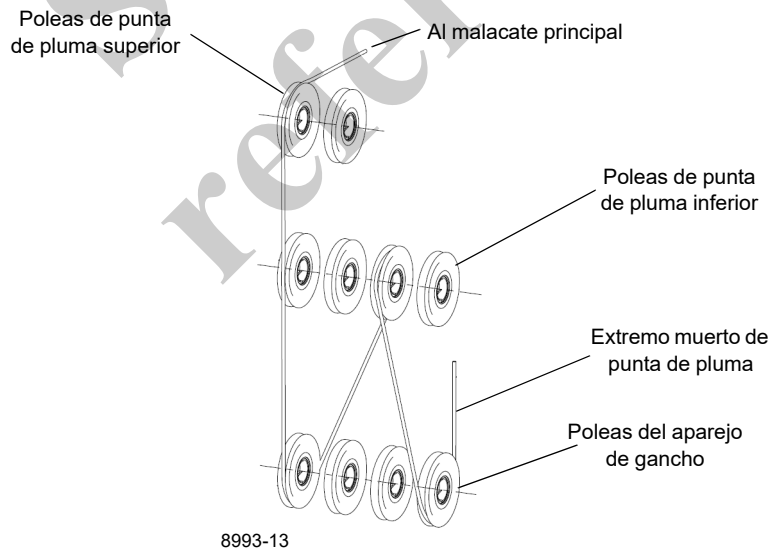
Cable de 4 secciones, aparejo de gancho con 4 poleas
