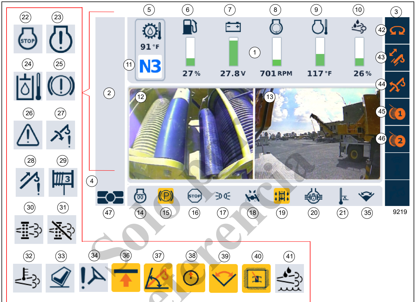
Vista de menú principal con el sistema de cámara de 3 vistas
