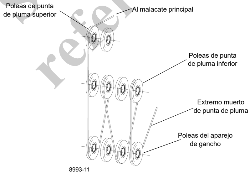
Cable de 6 secciones, aparejo de gancho con 4 poleas
