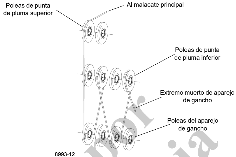
Cable de 5 secciones, aparejo de gancho con 4 poleas
