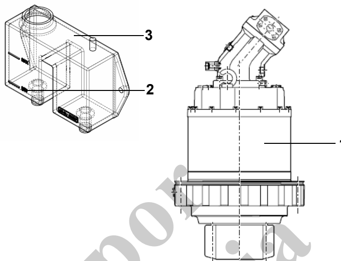
Fig. 241 Corona de giro y tanque de expansión de aceite
