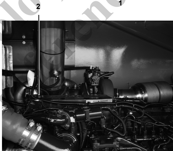
Fig. 205 Varilla de medición de aceite y cuello de llenado
