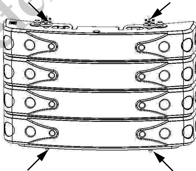
Fig. 221 Ubicación de las varillas de lastre con las tuercas hexagonales
