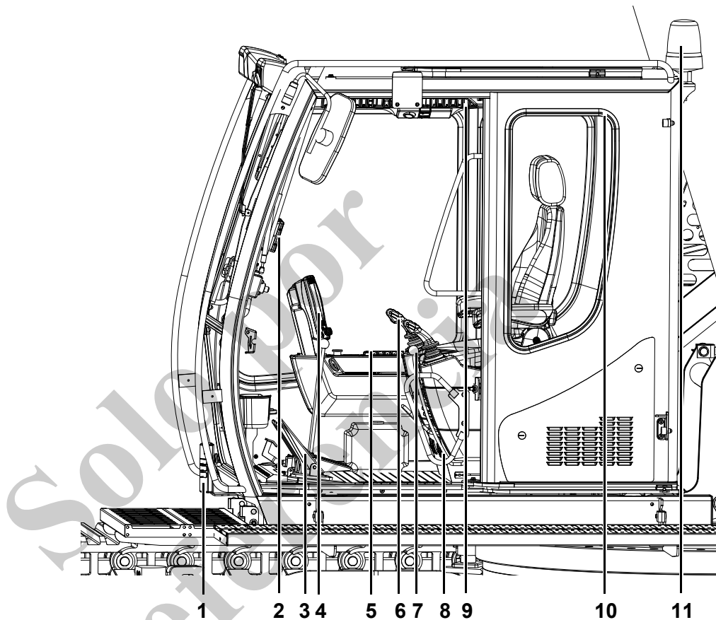
Fig. 59 Componentes de la cabina
