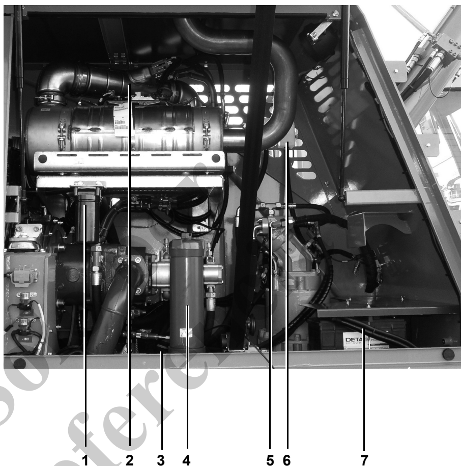
Fig. 17 Lado trasero derecho del compartimiento de motor
