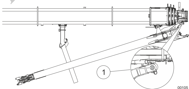
Fig. 153 Desempennado de la pluma de extremo de la cabeza de la pluma
