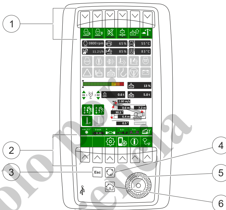
Fig. 22 Elementos de control del SENCON
