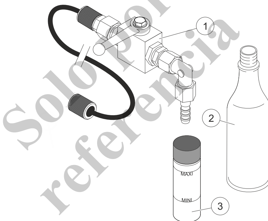
Fig. 250 Materiales para el muestreo del aceite hidráulico
