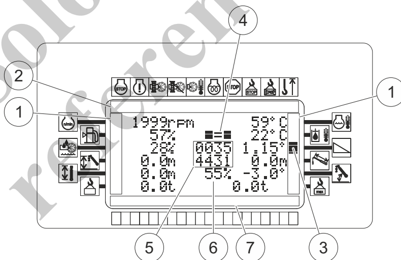
Fig. 80 Datos de motor mostrados en el control remoto por radio
