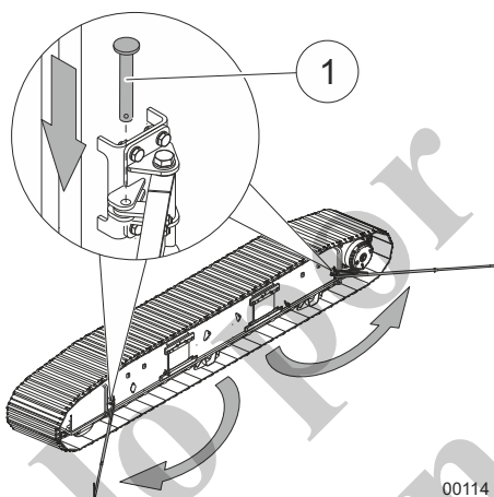
Fig. 129 Despliegado de la protección de la gama de giro
