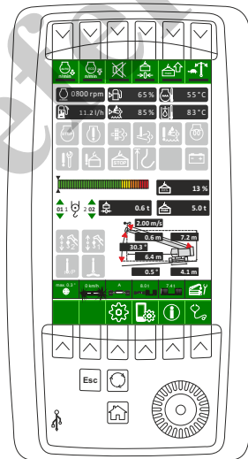
Fig. 197 Diagrama de trabajo
