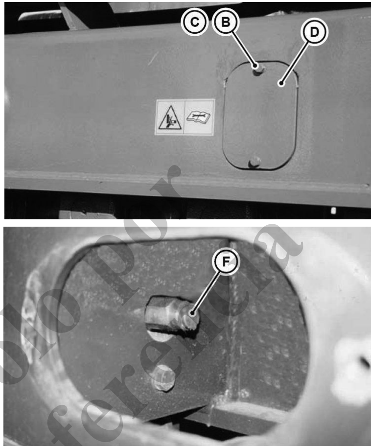
Fig. 226 Ubicación de la válvula de lubricación en el tren de rodaje
