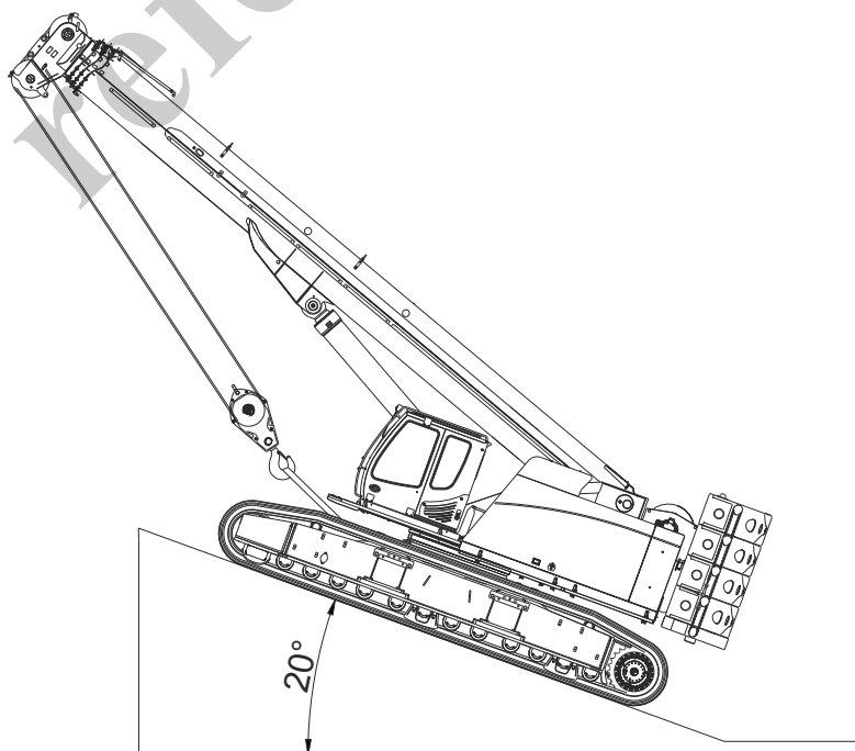
Fig. 85 Movimiento en terreno inclinado
