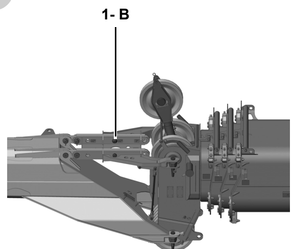
Pluma de extremo en la posición de 20°
