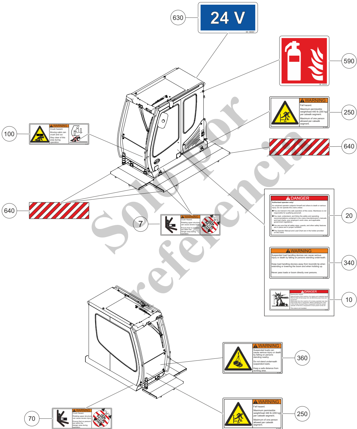
Fig. 5 Señalización de la cabina
