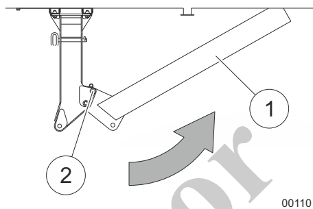
Fig. 168 Plegado y empernado de la rampa
