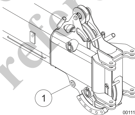
Fig. 147 Instalación de un cable para tirar de la pluma de extremo
