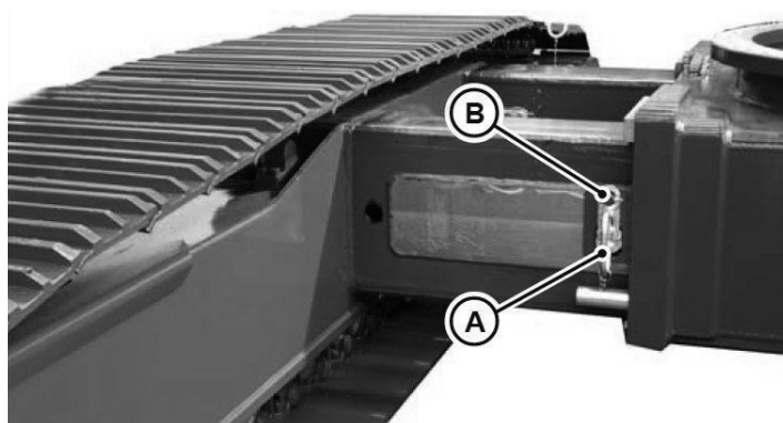
Fig. 106 Tren de rodaje con los pernos (A) y pasadores de pestillo (B) instalados
