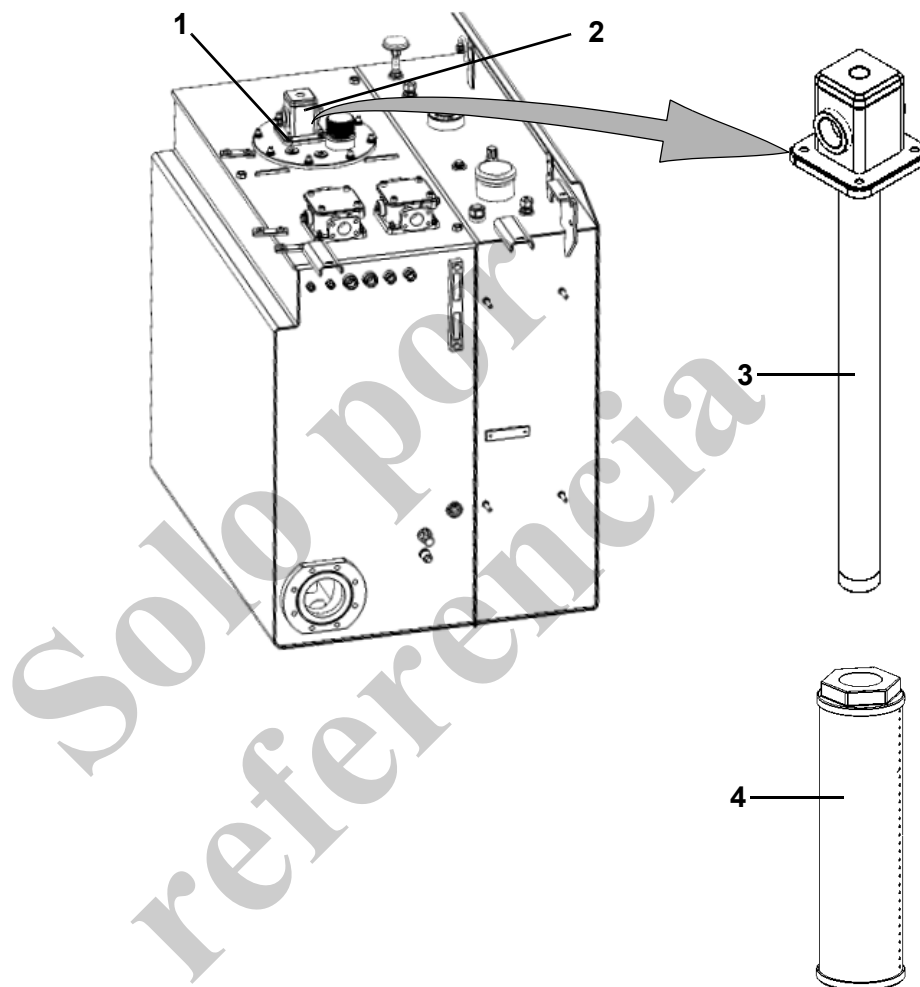
Fig. 216 Elemento de filtro de aceite de fugas en el tanque de combinación
