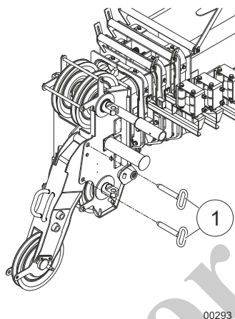
Fig. 186 Empenado del plumín auxiliar a la pluma telescópica
