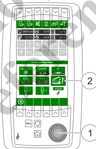
Fig. 20 Ventana del limitador del momento de carga en el SENCON
