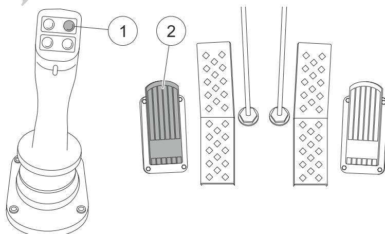
Fig. 87 Activación del giro libre de la corona de giro
