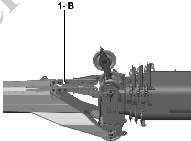
Pluma de extremo en la posición de 40°
