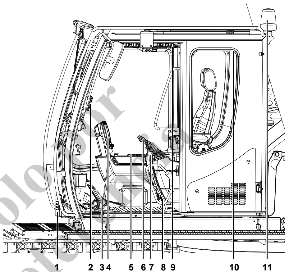
Fig. 14 Componentes de la cabina
