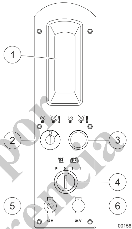
Fig. 65 Tablero de control derecho, cerca del asiento del operador
