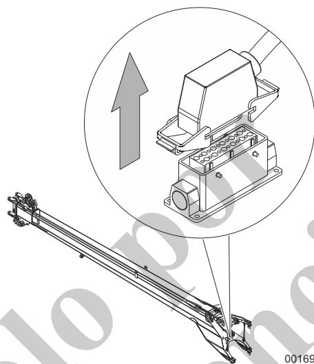
Fig. 140 Cable del interruptor limitador de elevación
