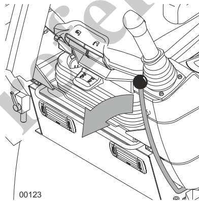
Fig. 199 Empujar la palanca de seguridad
