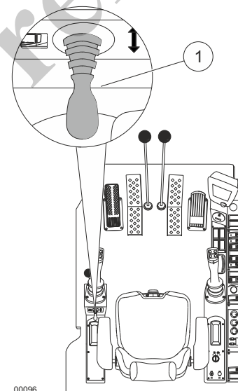
Fig. 58 Ajuste de la inclinación de la cabina
