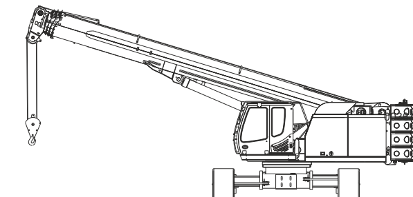
Fig. 49 Riesgo de vuelco debido a tren de rodaje retraído
