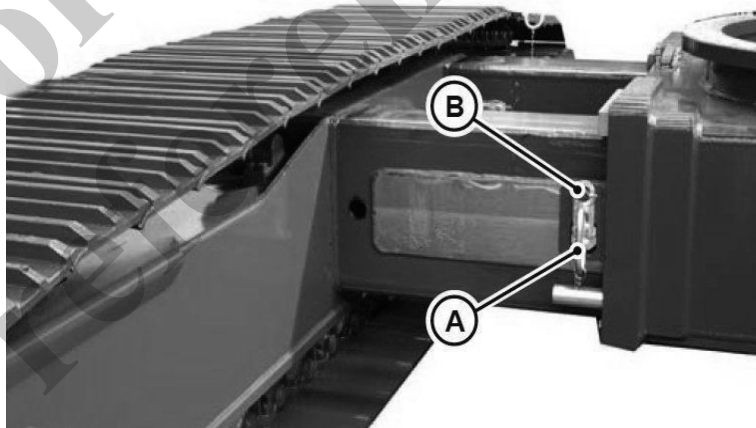
Fig. 107 Posición de los pernos (A) y de los pasadores de pestillo (B) en el tren de rodaje
