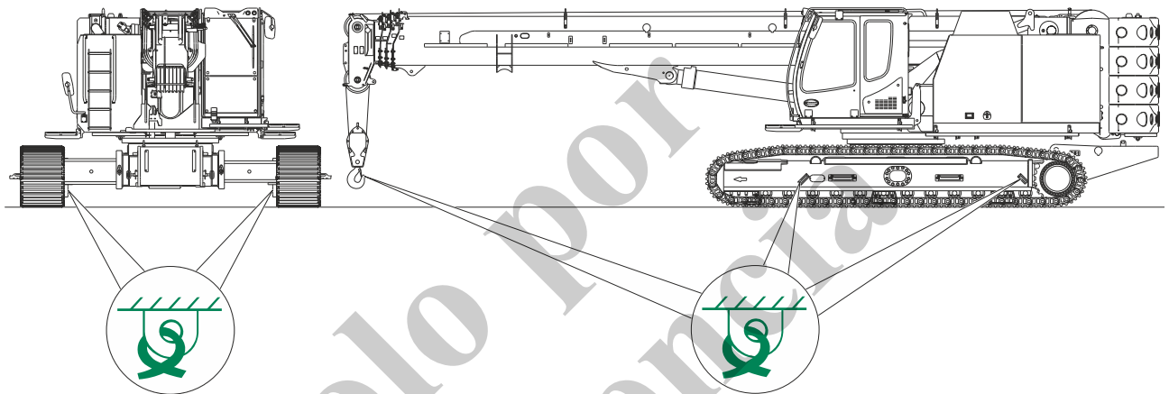
Fig. 201 Marca y posición de los puntos de sujeción
