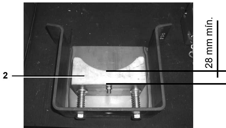
Fig. 237 Lubricación de la almohadilla de desgaste plástica deslizante del anillo de giro
