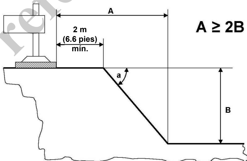
Fig. 1 Determinación de la distancia a terraplenes y excavaciones
