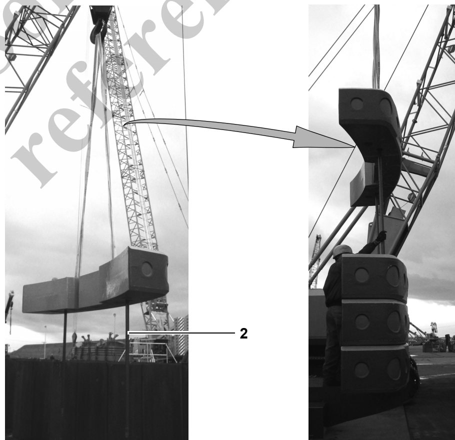
Fig. 121 Instalación del bloque de lastres superior con gancho en la varilla de lastre
