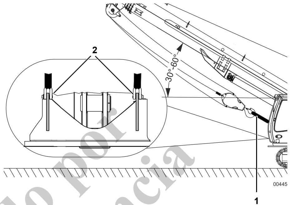
Fig. 84 Fijación del aparejo de gancho inferior para que no se mueva
