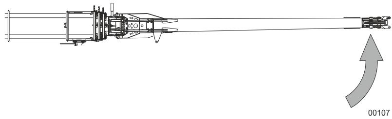
Fig. 165 Plegado de la pluma de extremo a la posición de trabajo
