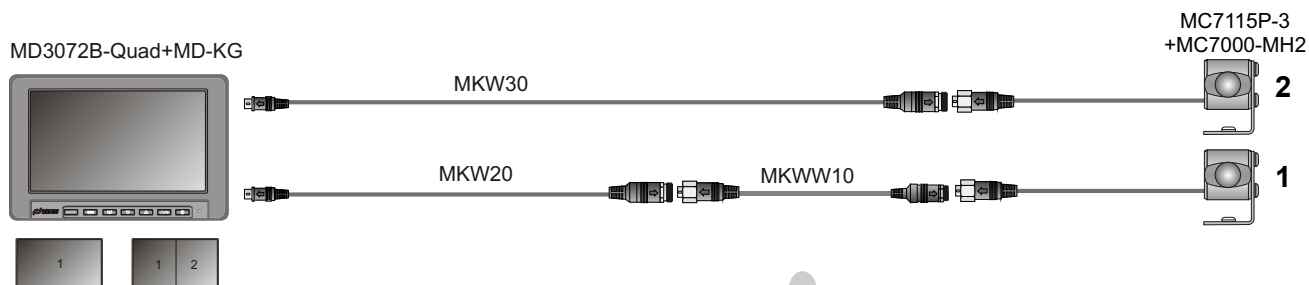
Fig. 70 Elementos del sistema de cámaras
