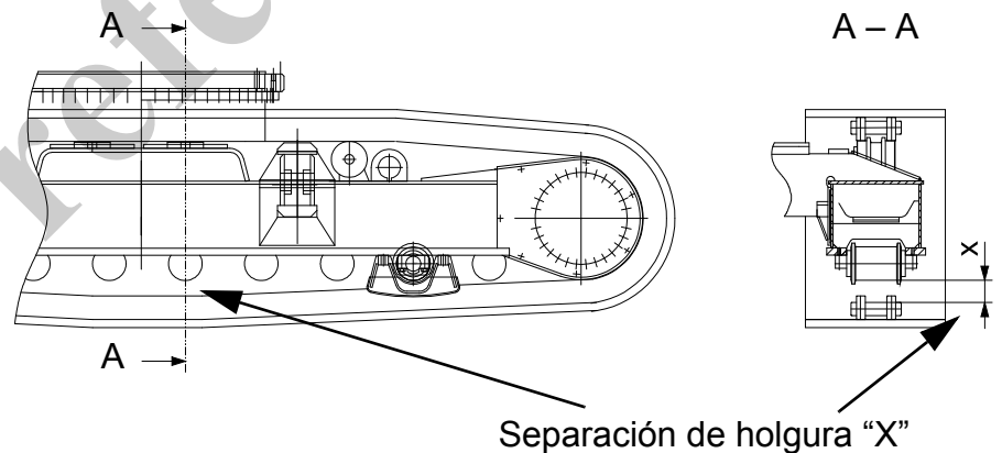
Fig. 230 Separación de holgura de la cadena de oruga
