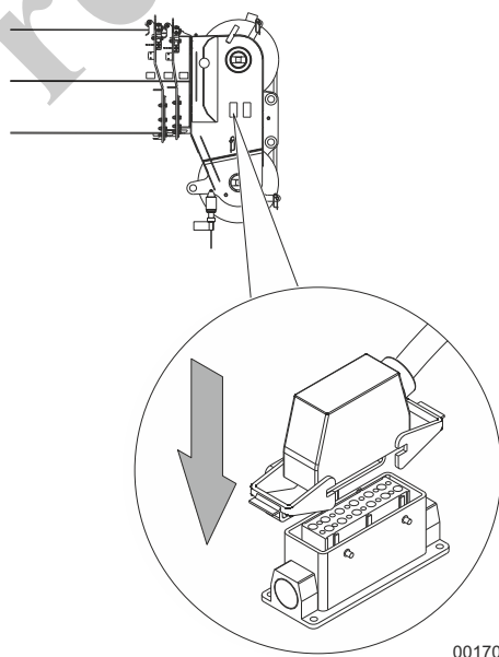
Fig. 141 Cable del interruptor limitador de elevación
