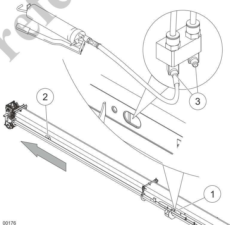
00176 Fig. 247 Lubricación de la pluma telescópica
