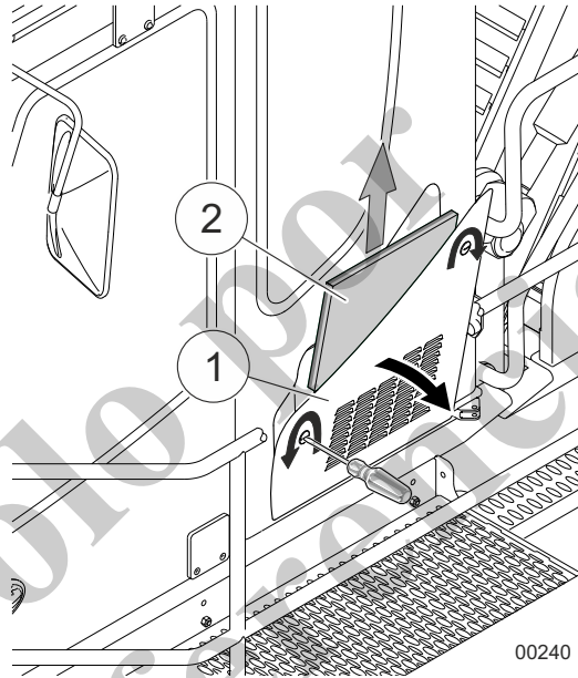
Fig. 246 Filtro de aire fresco
