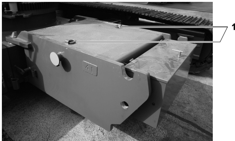
Fig. 110 Puntos de elevación en el lastre de tren de rodaje
