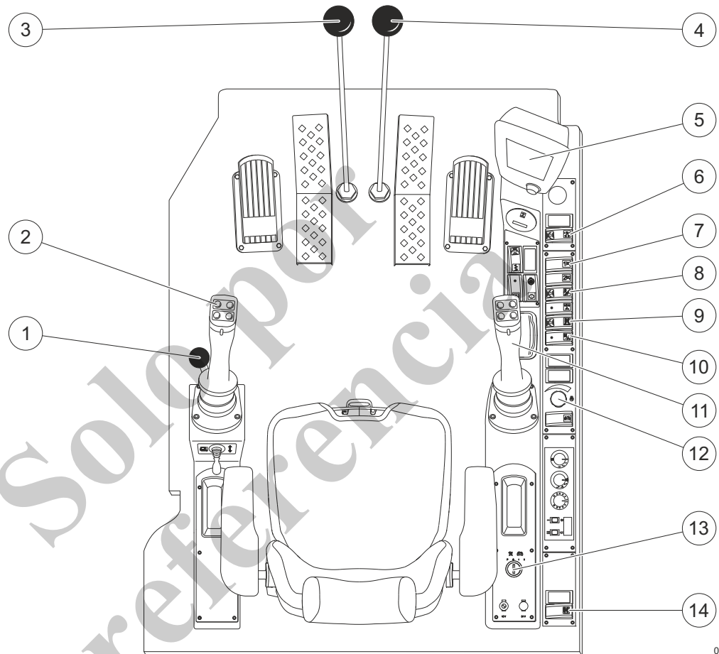
Fig. 191 Controles para descargar la máquina
