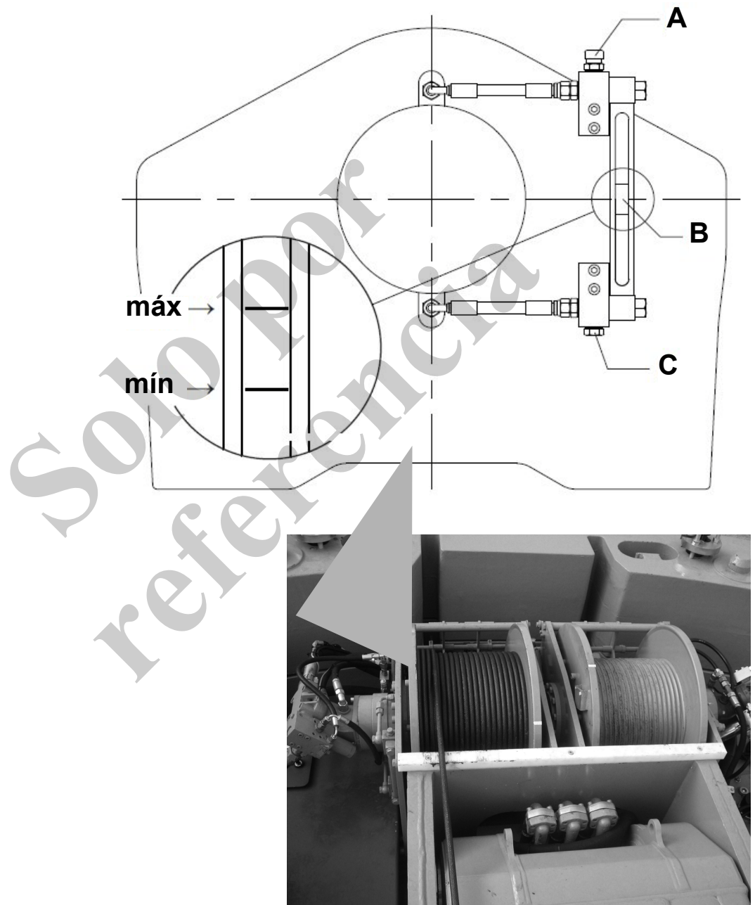
Fig. 220 Malacate
