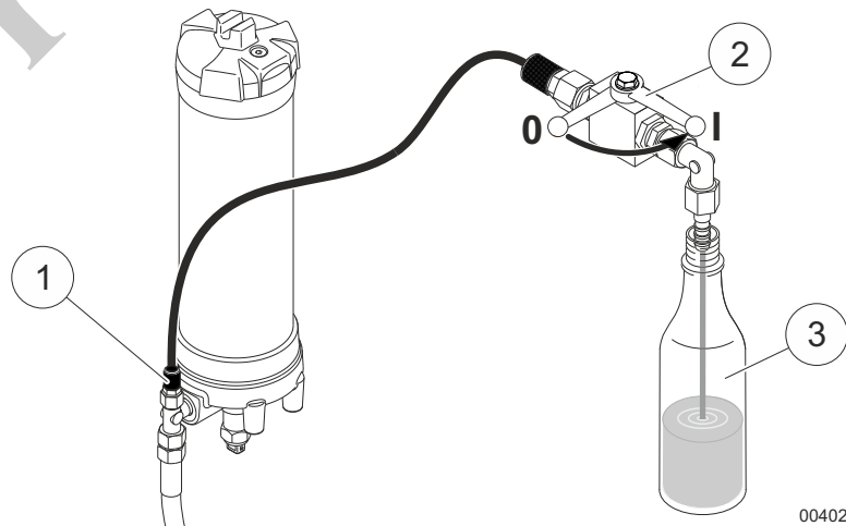
Fig. 251 Vaciado del aceite
