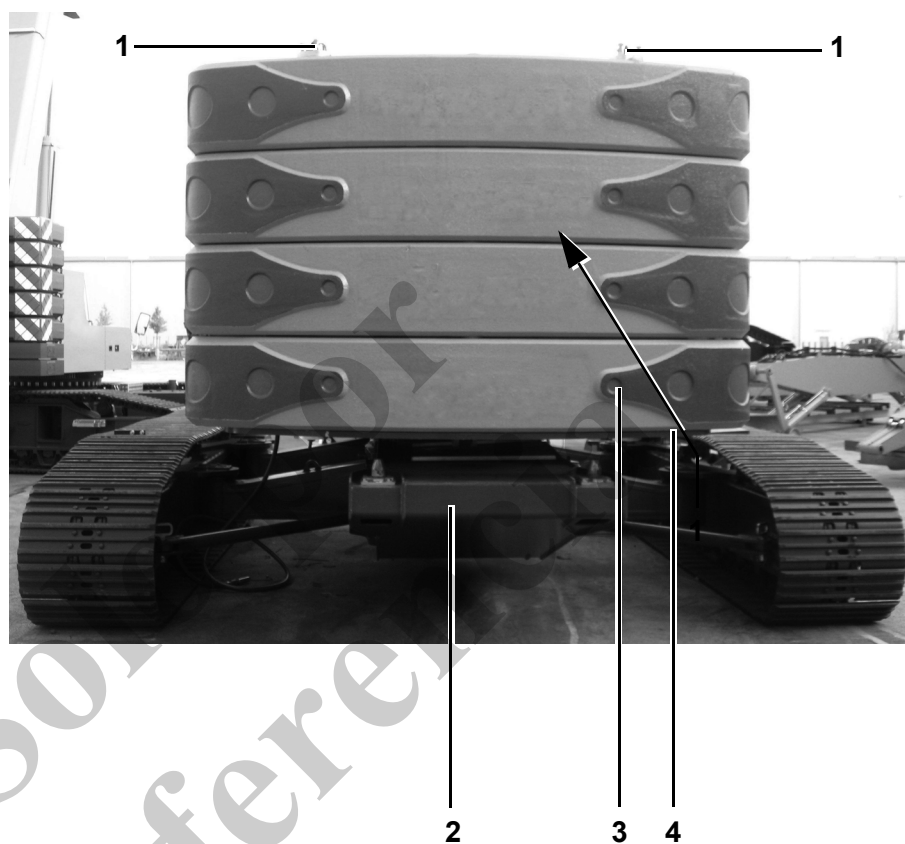
Fig. 22 Componentes del contrapeso
