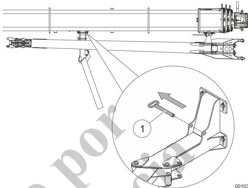
Fig. 161 Desempernado de la rampa
