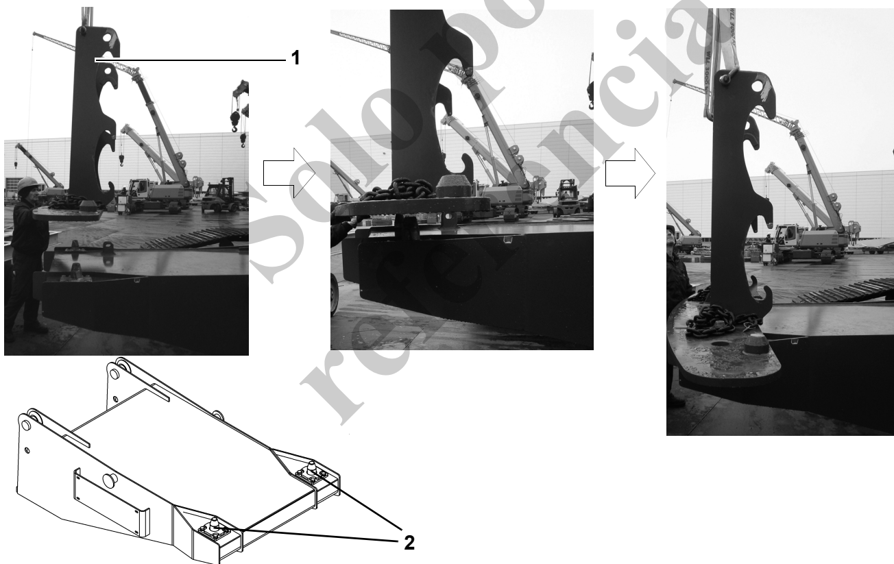
Fig. 118 Coloque el bloque de lastres en el soporte de lastres
