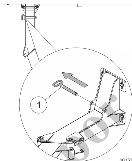
Fig. 148 Desempernado de la rampa
