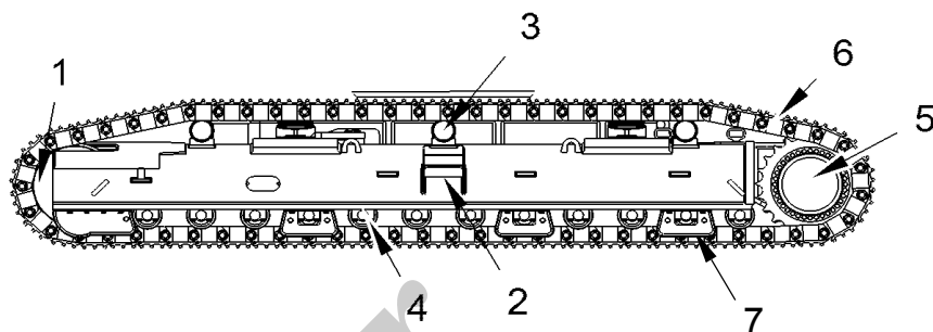
Fig. 13 Componentes del tren de rodaje
