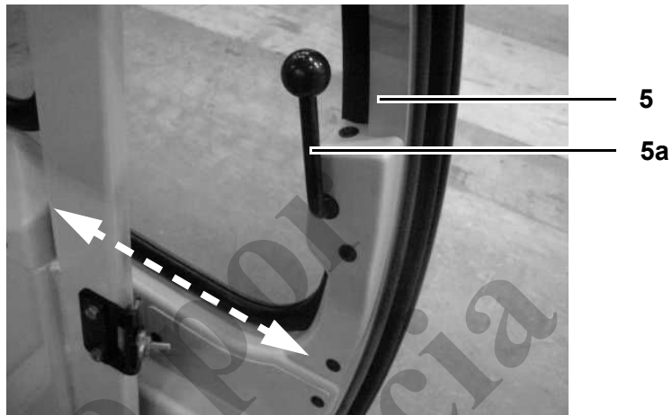
Fig. 51 Mecanismo de bloqueo de la puerta deslizante
