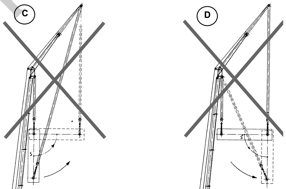
Fig. 91 Uso incorrecto del gancho con dos malacates
