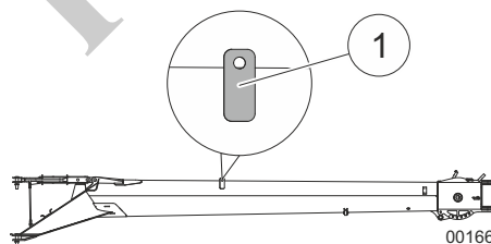
Fig. 135 Puntos de elevación de la pluma de extremo
