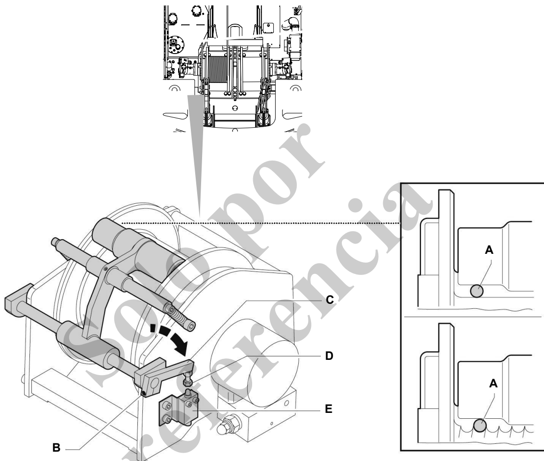
Fig. 76 Interruptor limitador de bajada en el malacate
