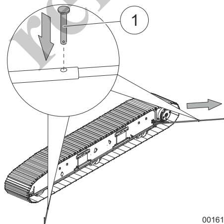
Fig. 130 Extracción de la protección de la gama de giro
