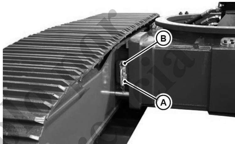
Fig. 103 Posición de los pernos (A) y de los pasadores de pestillo (B) en el tren de rodaje
