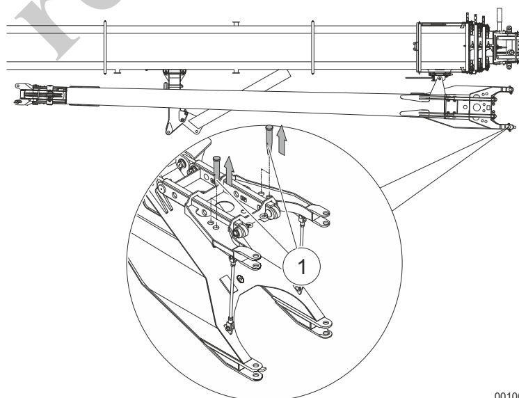
Fig. 157 Extracción del perno de la pluma de extremo
