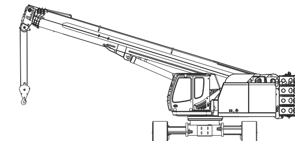
Fig. 190 Riesgo de vuelco debido a tren de rodaje retraído
