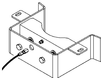
Fig. 236 Lubricación del patín plástico en el piñón
