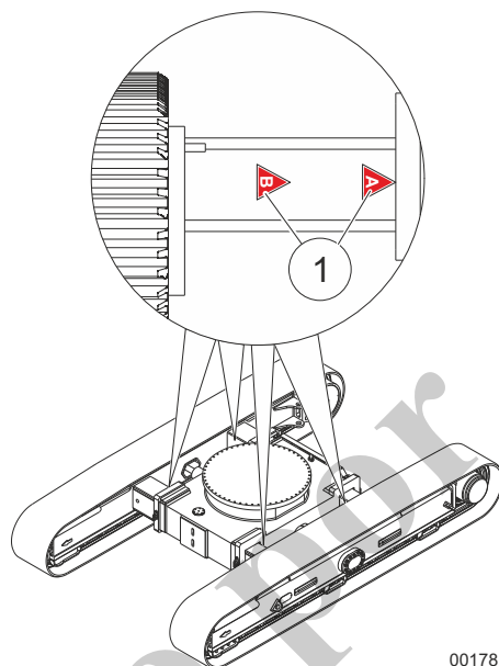
Fig. 102 Marca de ancho de vía con tren de rodaje totalmente extendido
