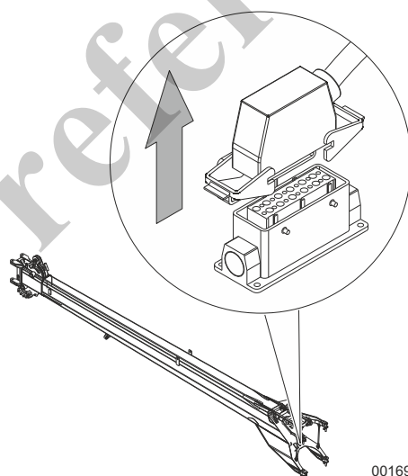
Fig. 169 Cable del interruptor limitador de elevación de la pluma de extremo
