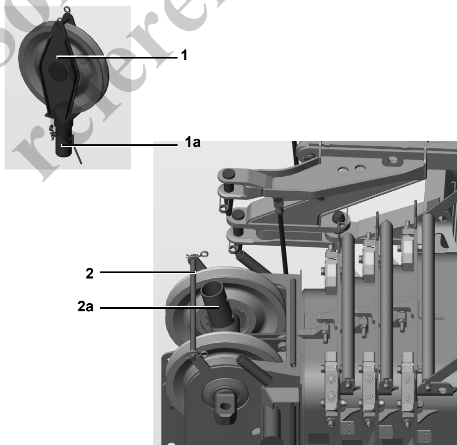
Fig. 133 Elementos de la polea de deflexión
