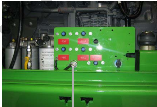
Fig. 244 Batería e interruptor de batería
