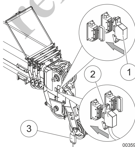
Fig. 187 Instalación del interruptor limitador de elevación del plumín auxiliar en la pluma telescópica
