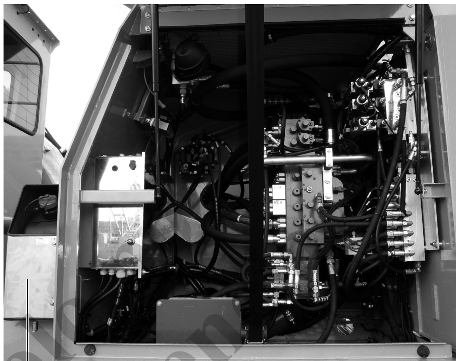
Fig. 99 Ubicación del depósito de DEF en la máquina
