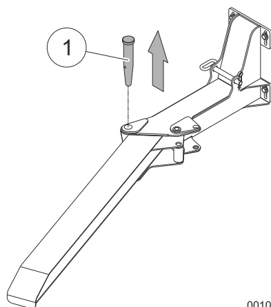
Fig. 167 Desempernado de la rampa
