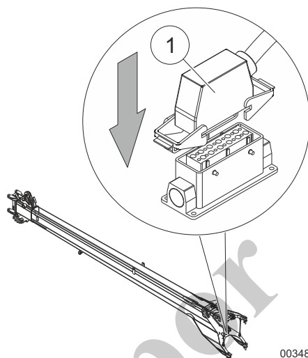
Fig. 142 Cable del interruptor limitador de elevación en la posición de estacionamiento
