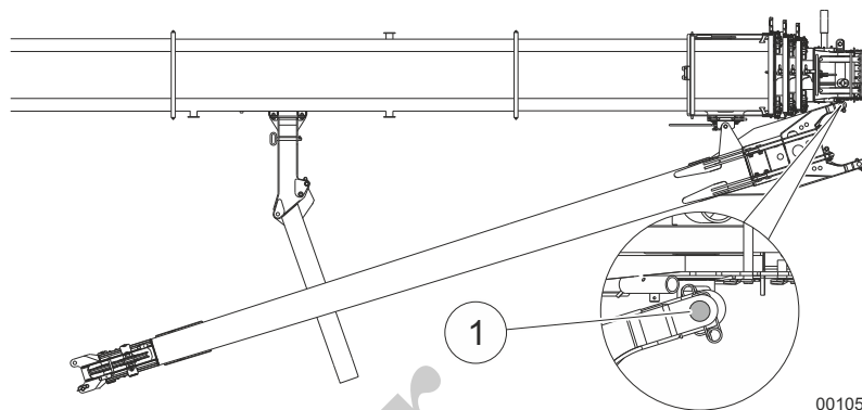
Fig. 163 Empenado de la pluma de extremo a la cabeza de la pluma
