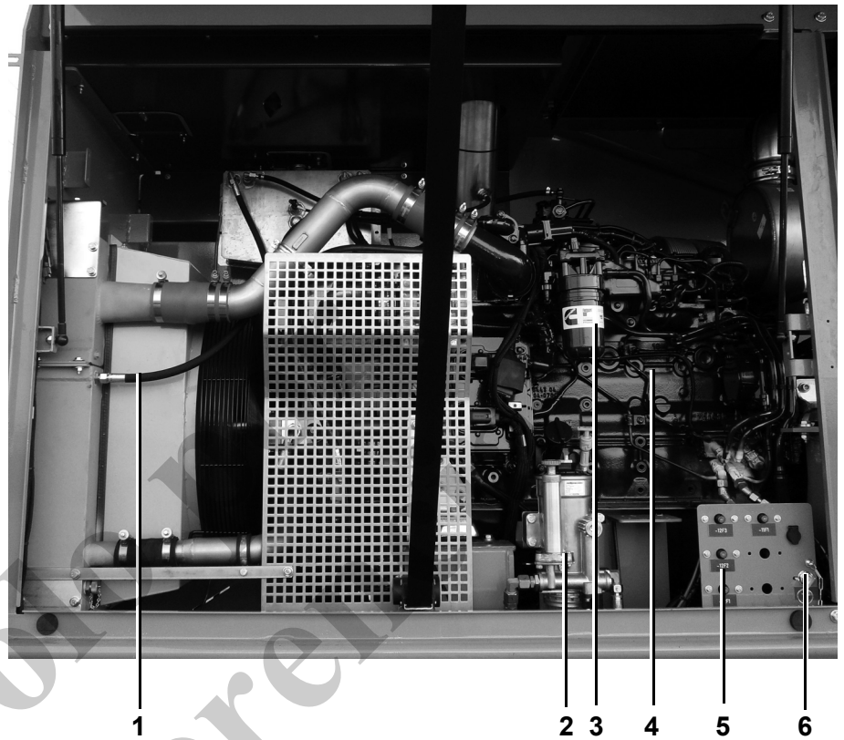
Fig. 16 Lado delantero derecho del compartimiento de motor
