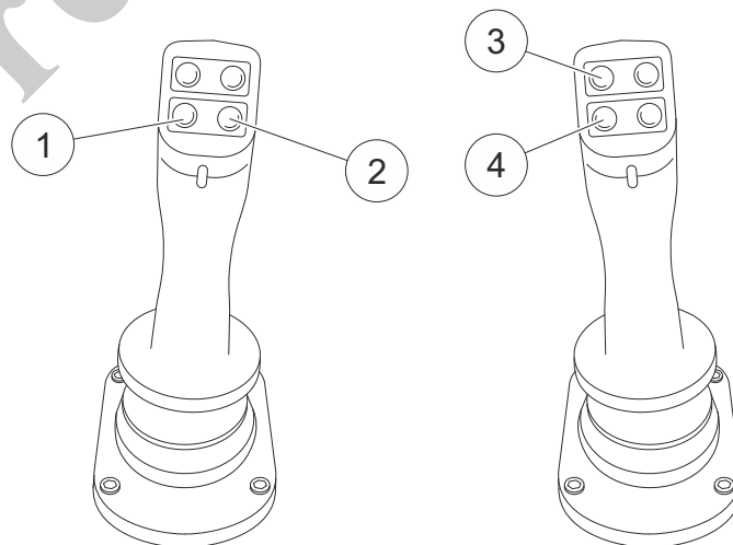
Fig. 94 Elementos de control para las tenazas de sujeción
