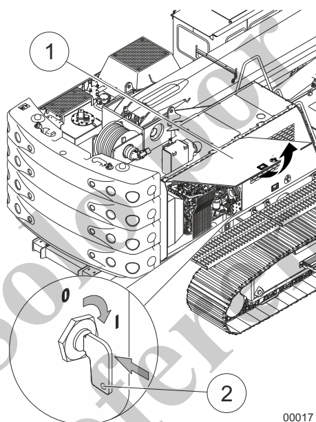
Fig. 14 Conexión del interruptor de la batería
