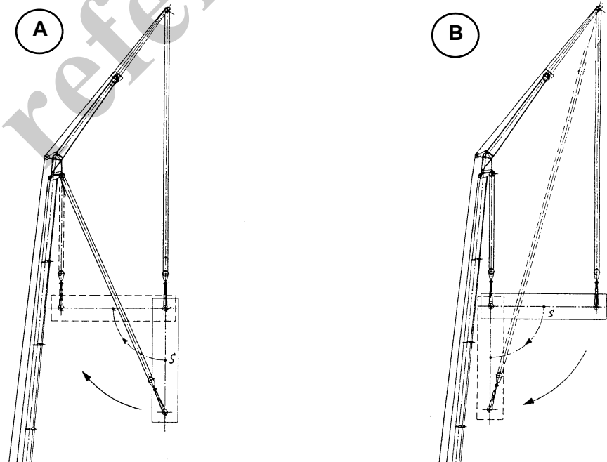
Fig. 90 Uso correcto del gancho con dos malacates
