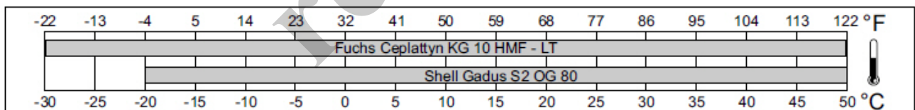
Fig. 11 Gamas de temperatura
