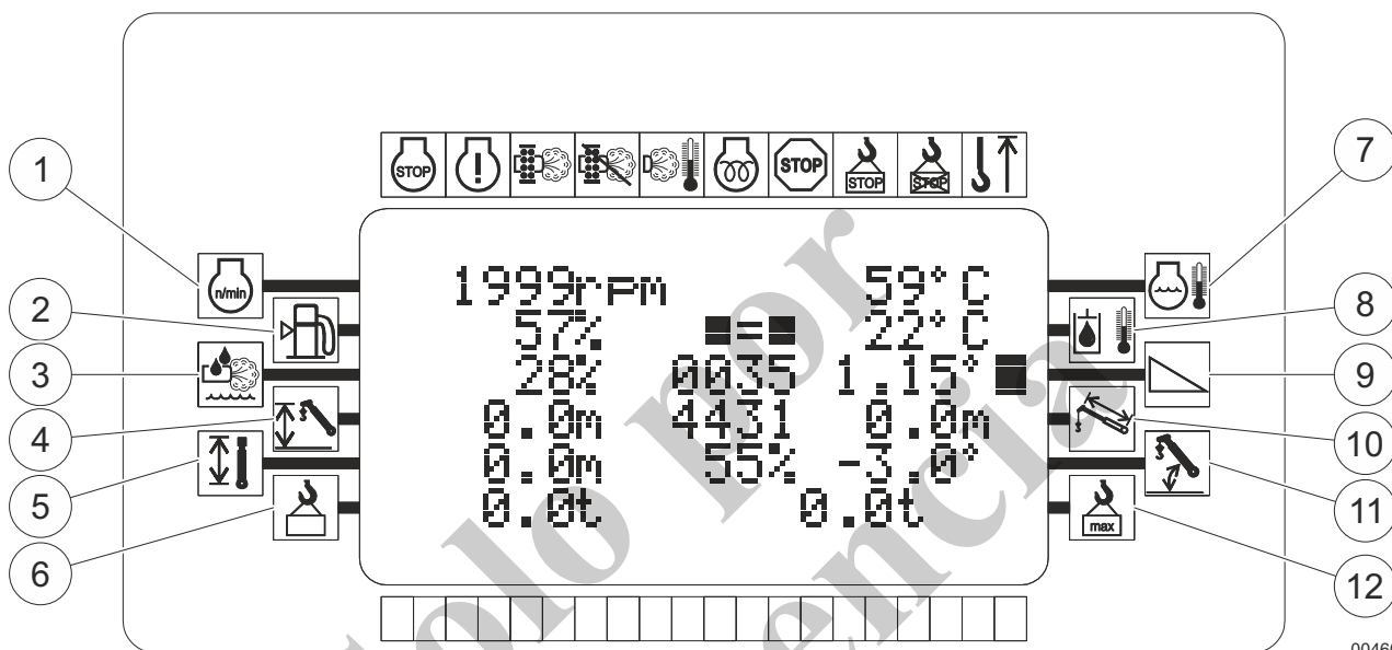
Fig. 81 Parámetros de funcionamiento mostrados en el control remoto por radio
