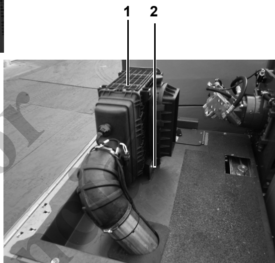
Fig. 206 Posición y elementos del filtro de aire
