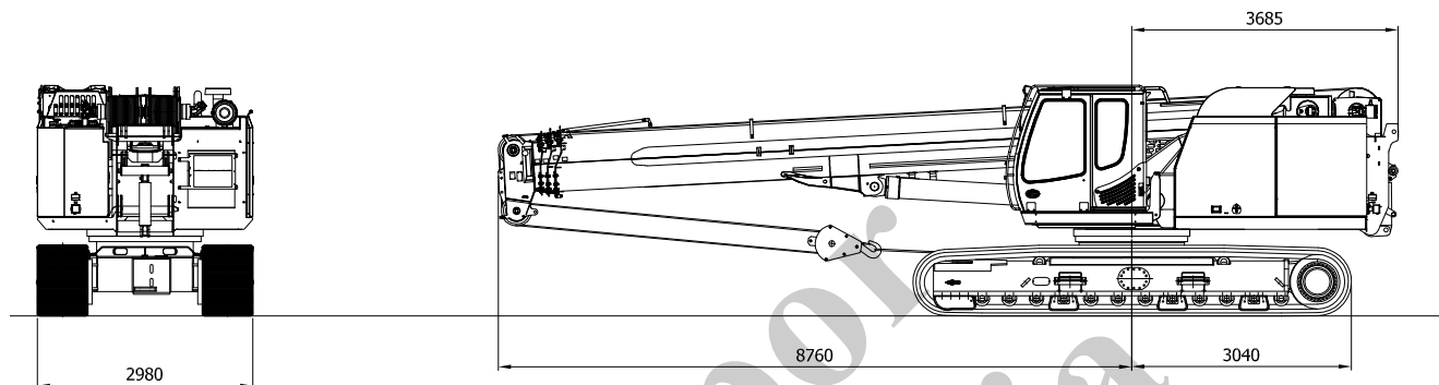
Fig. 202 Dimensiones de transporte de la máquina sin contrapeso
