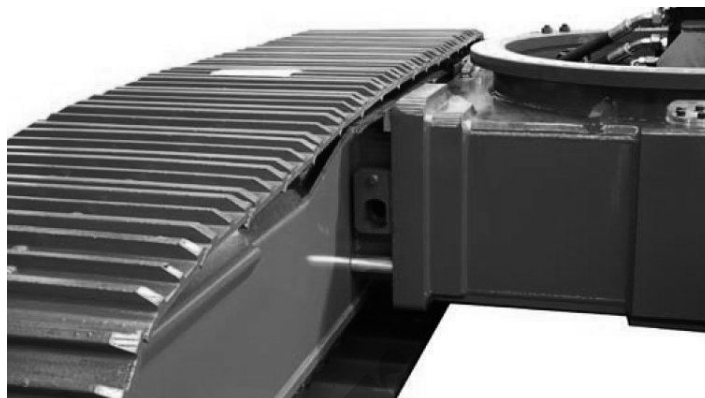
Fig. 104 Tren de rodaje con los pernos retirados
